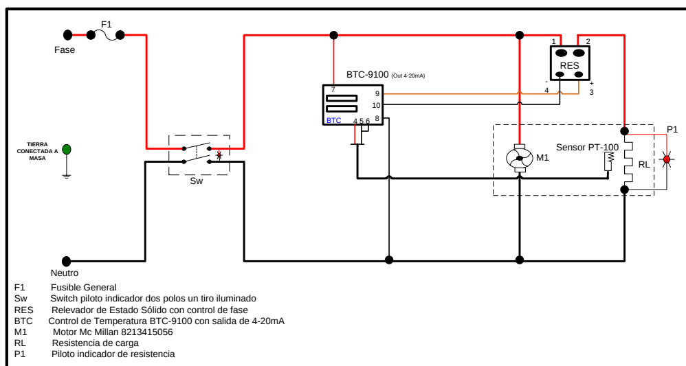
Diagrama de Control de Estufa Digital con motor TE-E35DM, TE-E45DM, TE-E61DM
