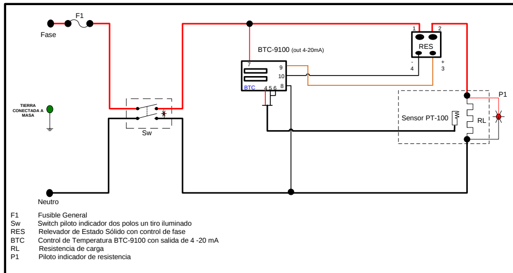
Diagrama de Control de Estufa Digital sin motor TE-E35D, TE-E45D y TE-E61D
