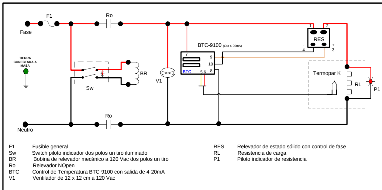
Diagrama de Control de Horno Digital sin motor TE-H218LD a 120 Vc.a.
