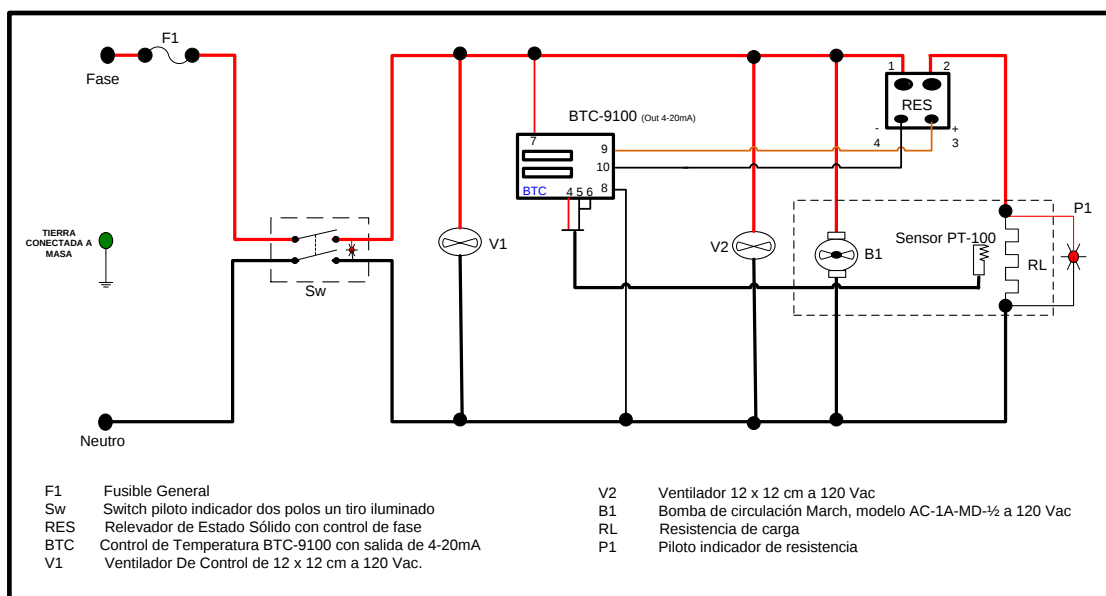
Diagrama de Control de Baño de Circulación TE-B40DC, TE-B80DC y TE-B160DC
