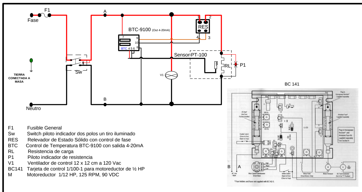
Diagrama de Control de Baño Digital de Movimiento Transversal TE-B160MT
