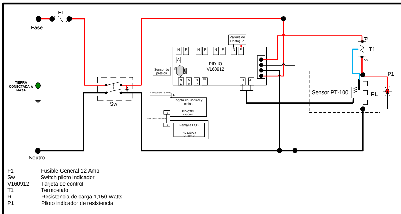
Diagrama eléctrico de Steam Bioclave
